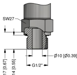
G1/2" DIN 3852 offener Anschluss, p_N \leq 40 bar
