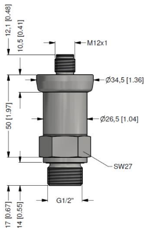
G1/2" DIN 3852 mit M12x1
