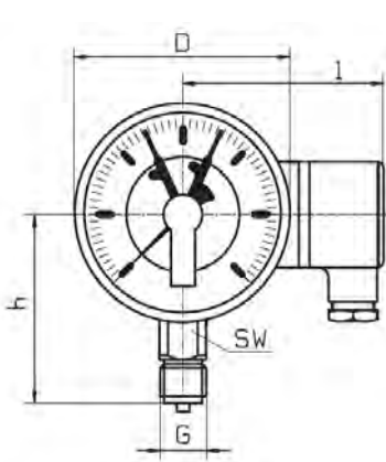
Anschluss unten
