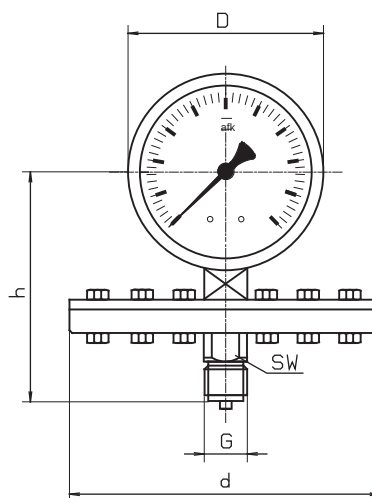
Flange 160 mm
