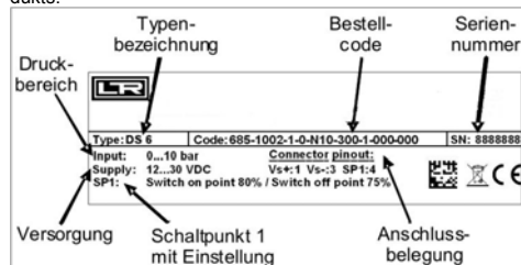
Abb. 1 Typenschild
