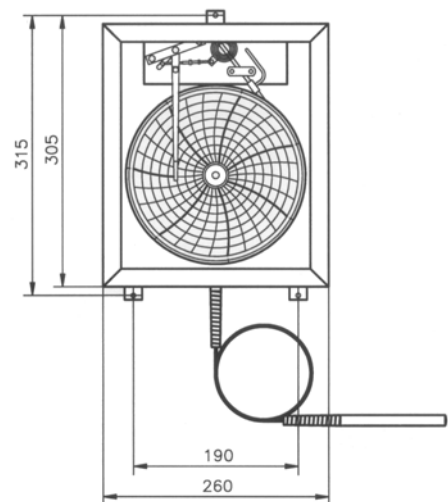
Bild 7 Kreisblattschreiber Typ 355
