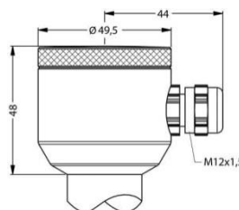
Kompakt-Feldgehäuse (IP 67)
