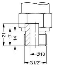
G1/2" offener Anschluss
