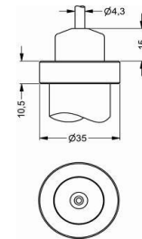
Kabelausgang mit PVC-Kabel (IP 67) 5
