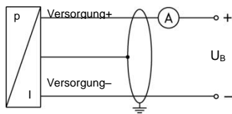
2-Leiter-System (Strom)
