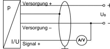
3-Leiter-System (Strom / Spannung)
