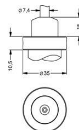
Kabelausgang, Kabel mit Belüftungsschlauch (IP 68) 6
