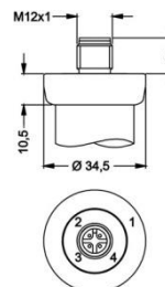
M12x1 4-polig (IP 67)
