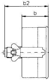
Type 097.4 Anschluss zentrisch hinten mit Klemmbügelbefestigung zum Schalttafeleinbau Centric back connection with u-clamp for panel-mounting
